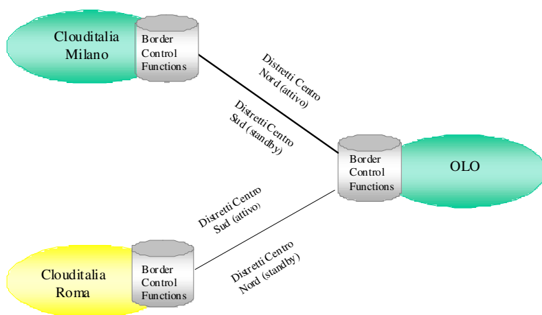
Figura 2 Modello architetturale d'interconnessione
